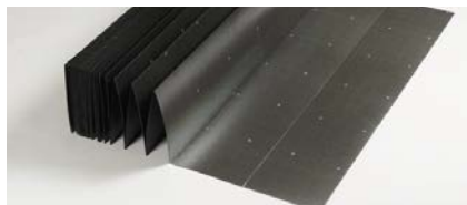
Solid-Protect Especial para vinilo de material macizo con una resistencia a la compresión de hasta 50 000 kg/m 2 Grosor: 1 mm
