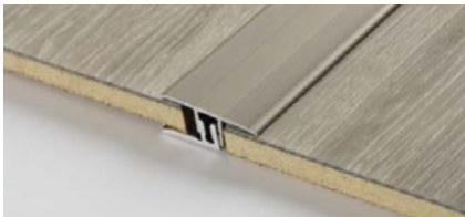
Perfil de transición aluminio de plata anodizada / acero fino
